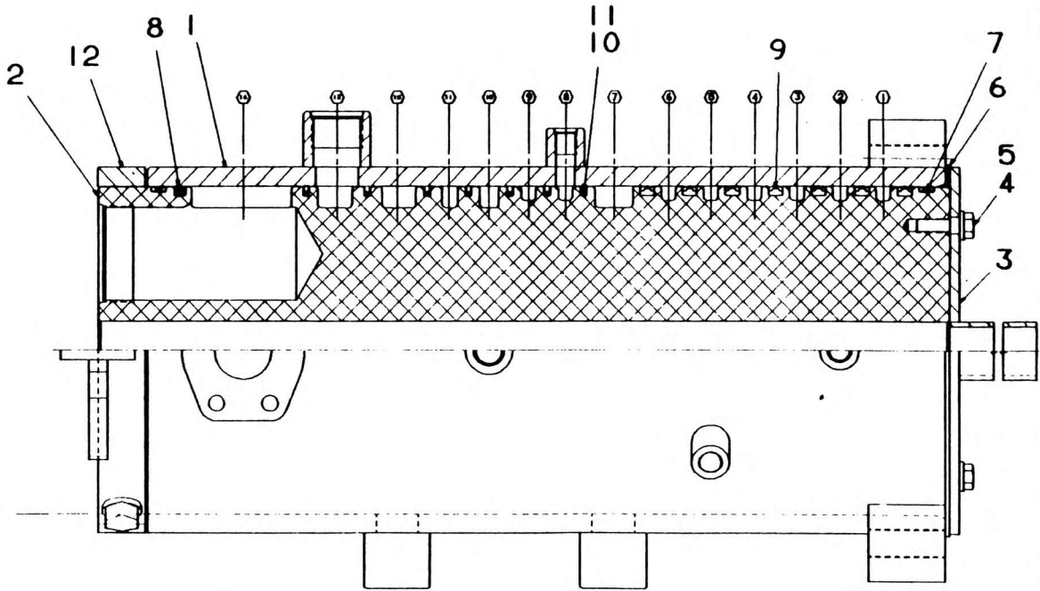
SECTION A-A
